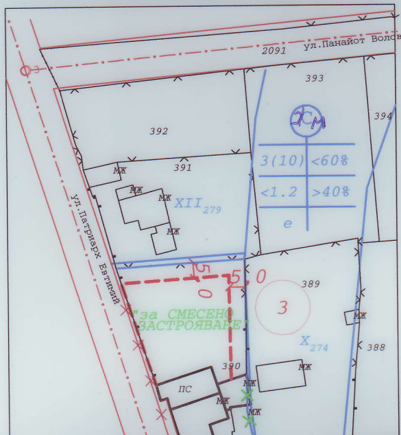
ПЛАН ЗА ЗАСТРОЯВАНЕ на УПИ ХІ-280, кв.3 на гр. Дългопол, общ. Дългопол, обл. Варна
